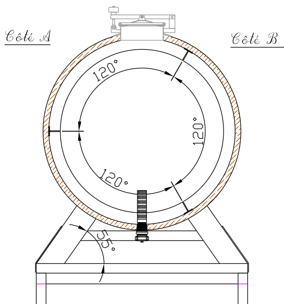
Vue en coupe transversale
