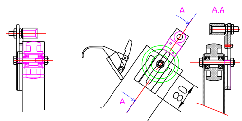
Détails châssis (1/10)
