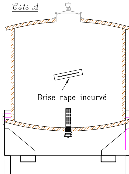
Vue en coupe longitudinale
