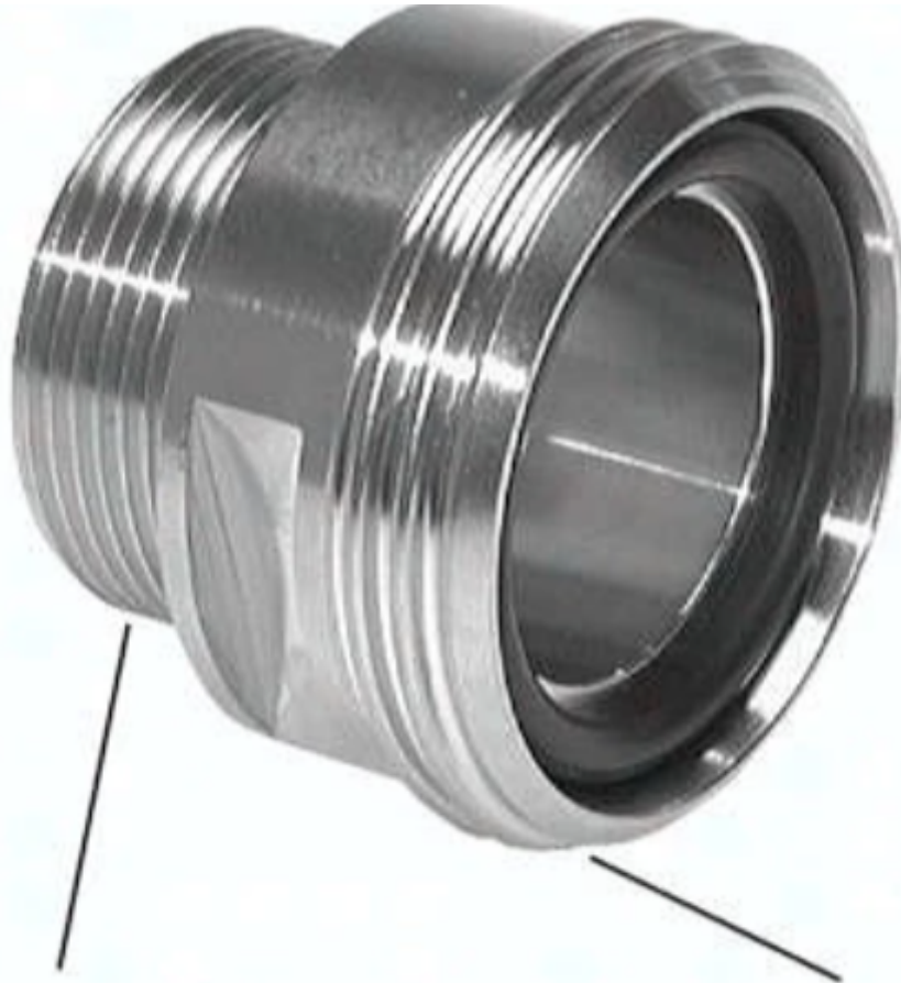
Gwint DIN 11851
